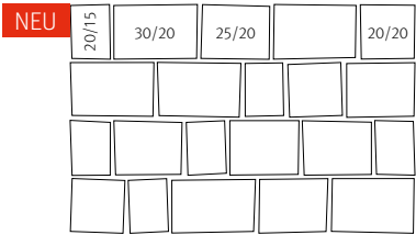
Großpflastersystem (Typ BI)
