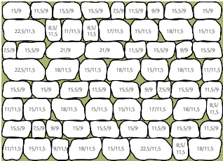
Kleinpflastersystem (Typ BH) Dicke 8 cm
