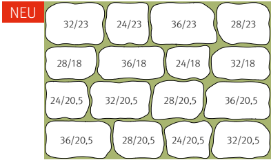
Großpflastersystem (Typ BK) Dicke 8 cm
