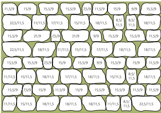
Kleinpflastersystem (Typ BF) Dicke 10 cm
